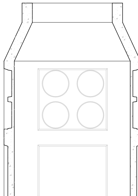
SECCIÓN B-B'
