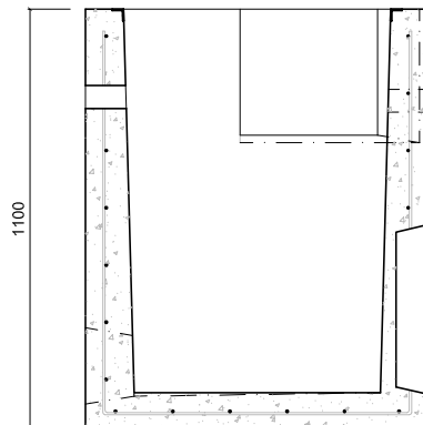
Sección B-B'
