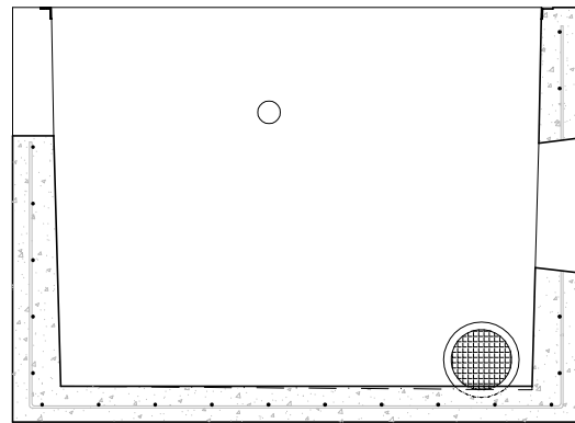
Sección A-A'
