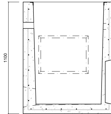
Sección B-B'
