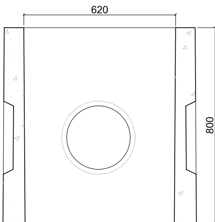
Sección A-A'
