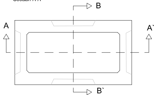
Sección A-A'
