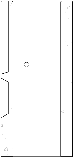
Sección B-B'
