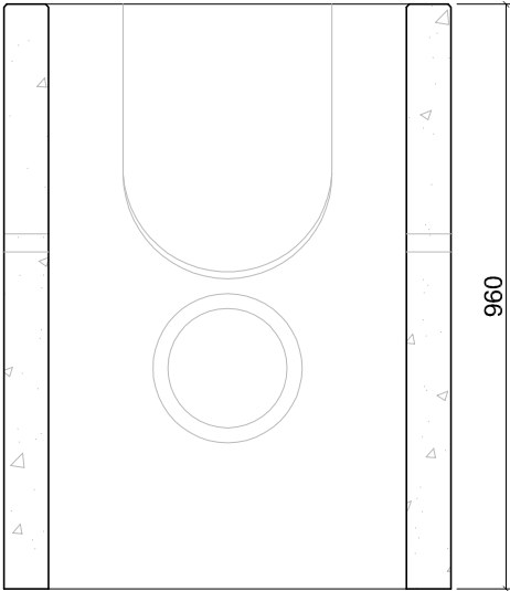
Sección A-A'
